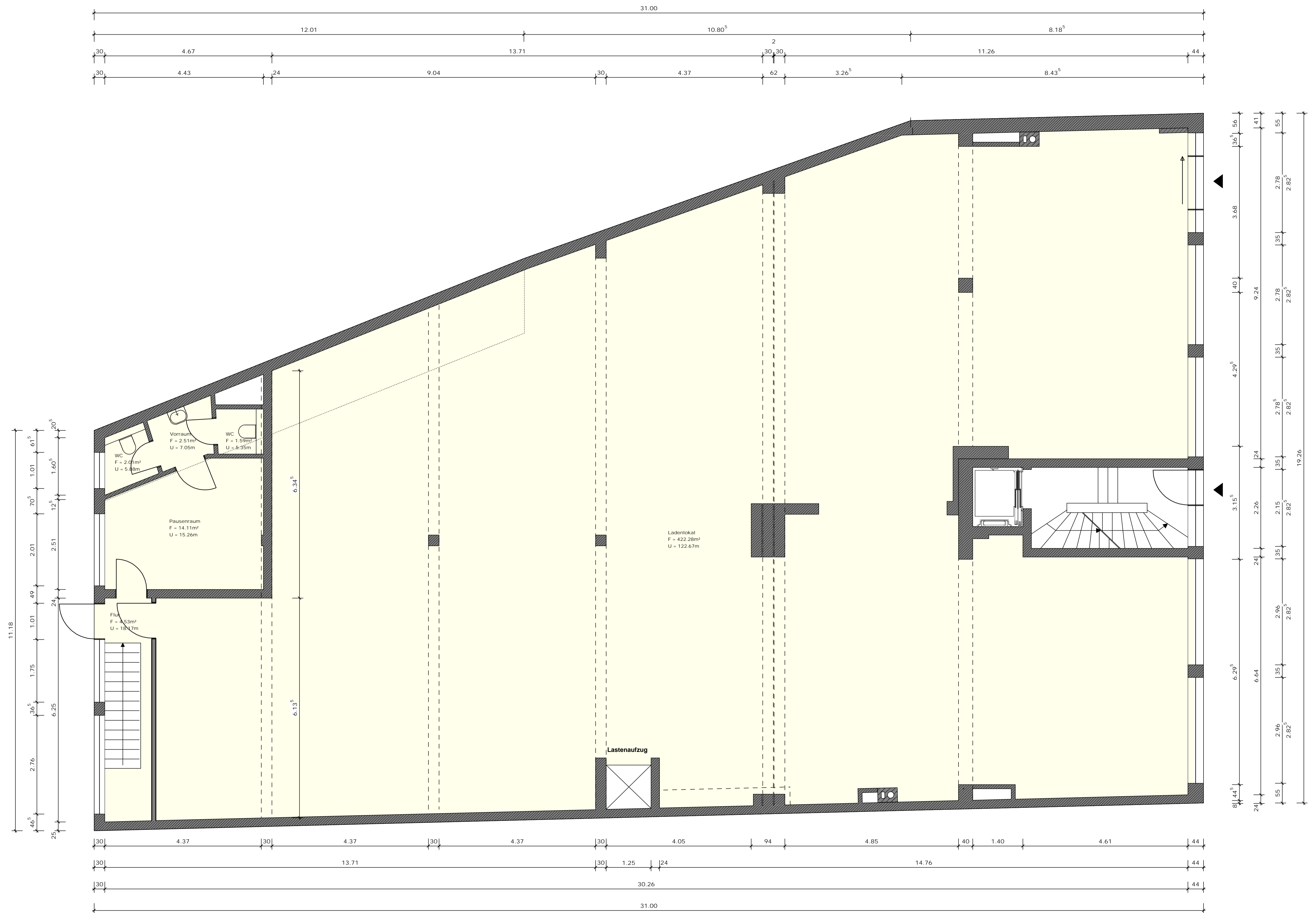
Grundriss Erdgeschoss
